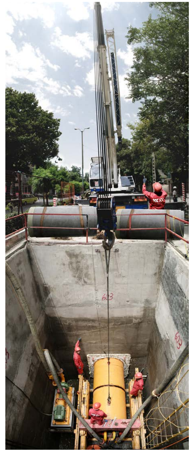
مشروع الصرف الصحي همدان على طريقة سحب الانبوب (منجز)
