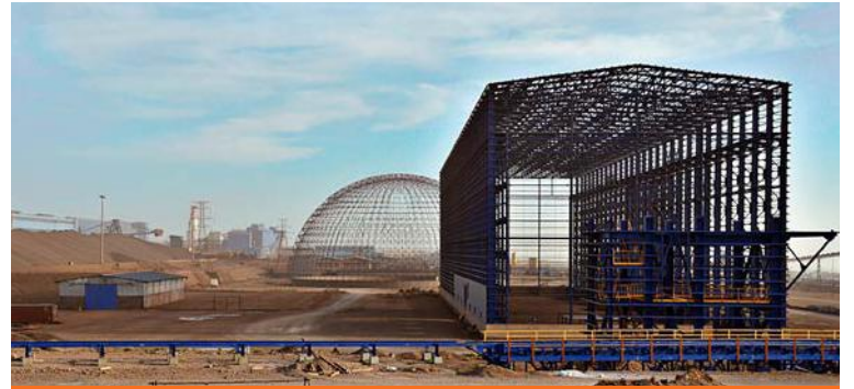
مصنع حجر الديد سنجان ( قيد التنفيذ )
